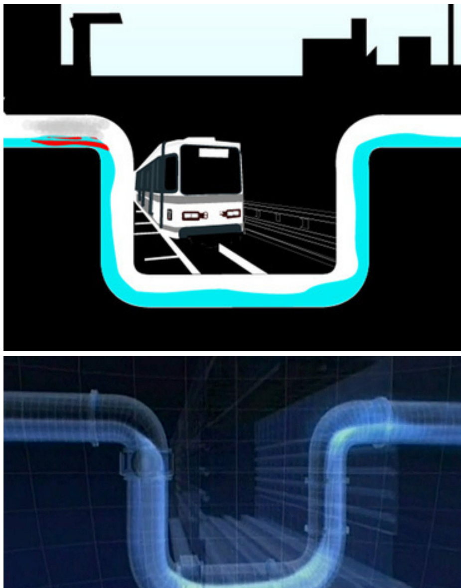
Сн. 10 и 11 Техническото решение за преодоляване на канализацията от тунела на метрото
