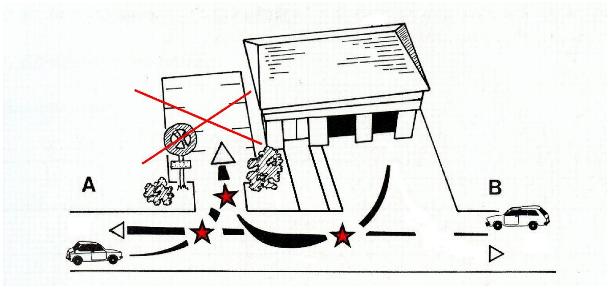
Фиг. 2. Пример за конфликтни точки при неправилно разполагане на паркинга за лични МПС. В случая конфликтните точки са три - наблюдава се пресичане на пътния поток
