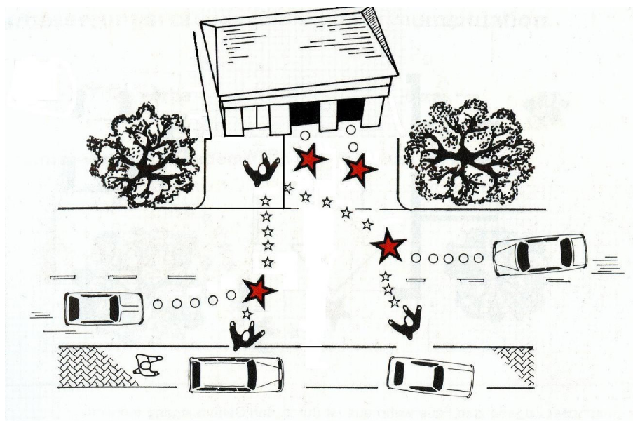
Фиг. 5. При паркиране в близост до пожарната служба – в случая на отсрещния тротоар, възникват четири конфликтни точки: две на пътя и две пред самите гаражни клетки
